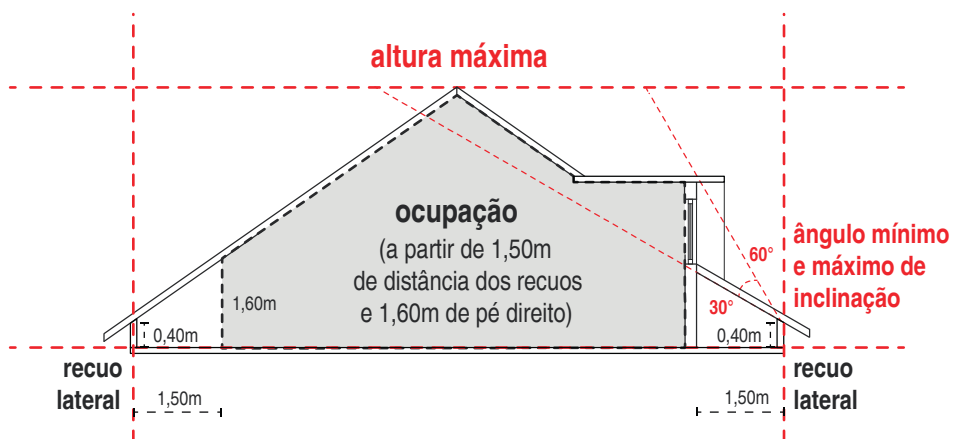
Fig. 11. Subtelhado
