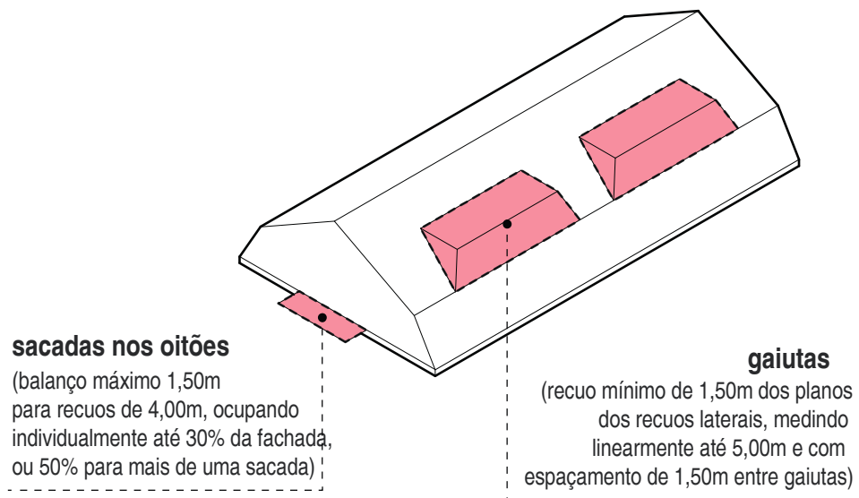
Fig. 10. Sacadas e gaiutas
